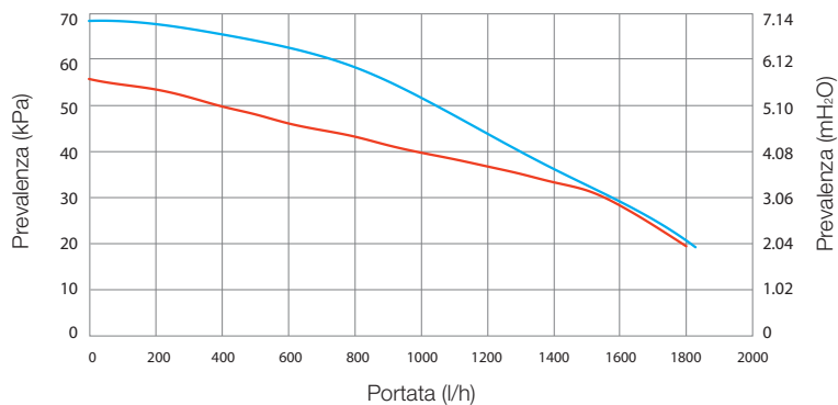
Grafico portata e prevalenza
