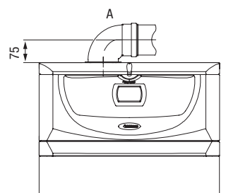
Quota kit concentrico Ø 60/100
