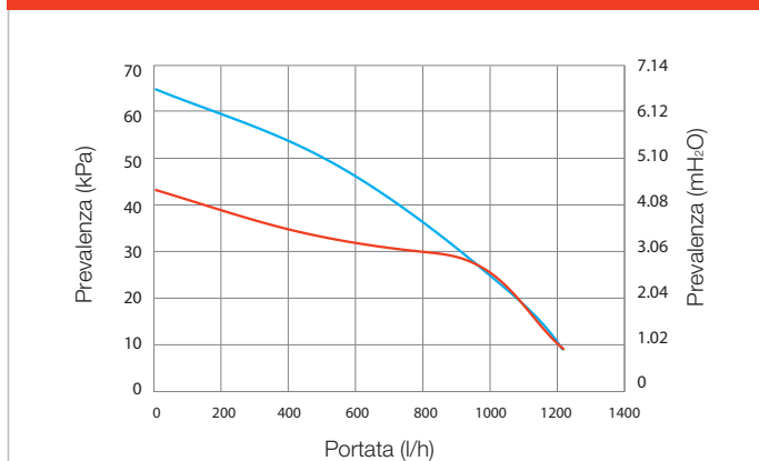
Grafico portata e prevalenza VICTRIX 26 kW/Plus
