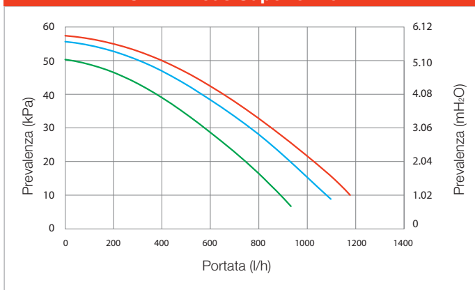
Grafico portata e prevalenza VICTRIX Zeus Superior 26 kW
