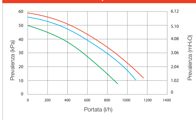
Grafico portata e prevalenza VICTRIX Superior 26 kW
