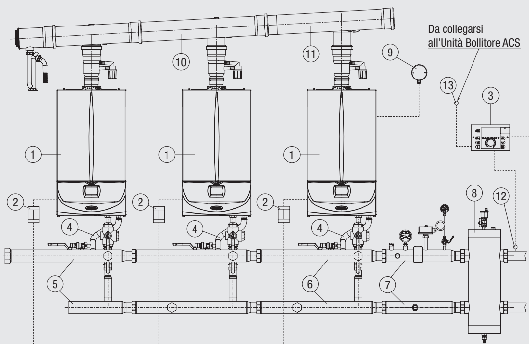
Schema idraulico d'installazione di 3 VICTRIX Superior 32 kW Plus in cascata
