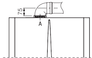
Quota kit concentrico Ø 60/100
