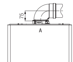
Quota kit concentrico Ø 60/100
