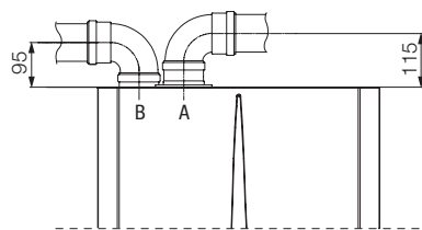
Quota kit separatore Ø 80/80
