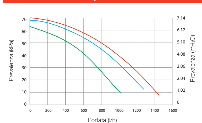
Grafico portata e prevalenza VICTRIX Superior 32 kW/Plus
