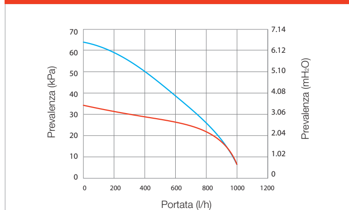
Grafico portata e prevalenza VICTRIX 12 kW X
