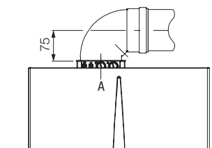
Quota kit concentrico Ø 60/100
