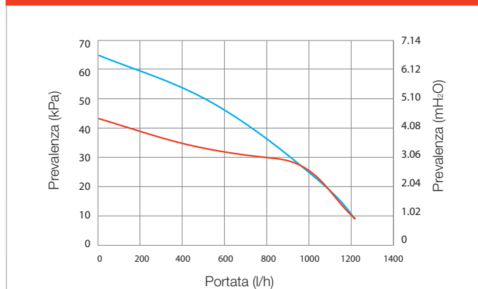
Grafico portata e prevalenza VICTRIX 26 kW/Plus
