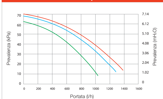
Grafico portata e prevalenza VICTRIX Zeus Superior 32 kW
